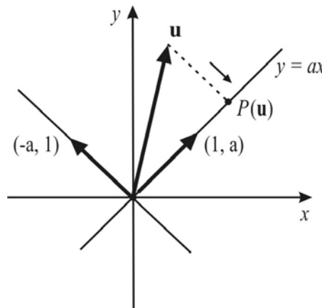
Figura 3.3: Projecção de um vetor \mathbf{u} \in \mathbb{R}^2 sobre a reta y = ax .
